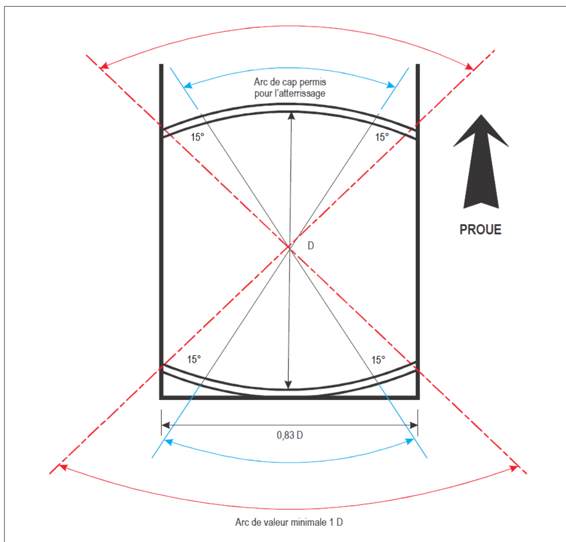
Figure 3-10. Caps d'atterrissage autorisés à bord des hélisations sur navire pour des opérations avec a cap limité
