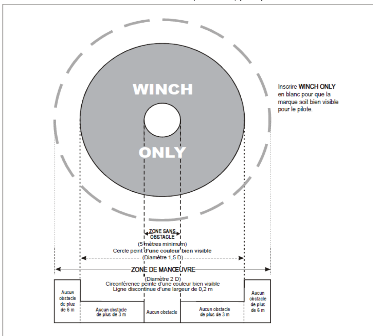
Figure 4-12. Aire d'hélicreusement d'un navire
