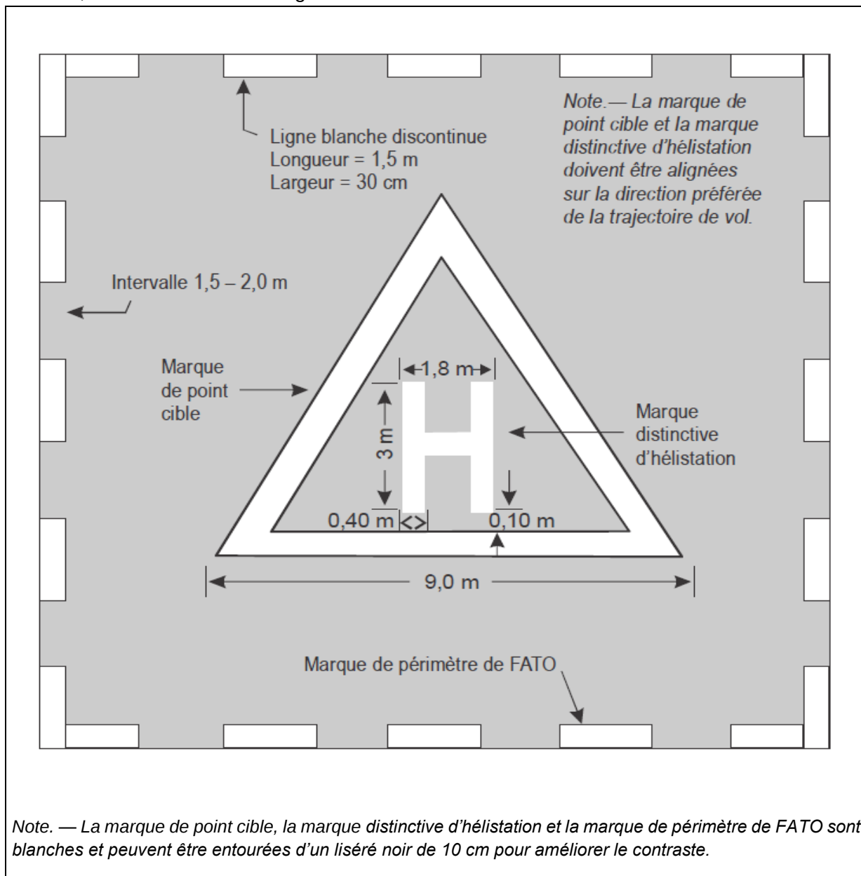
Figure 5-1. Combinaison de la marque distinctive d'hélistation, de la marque de point cible et de la marque de périmètre de FATO
